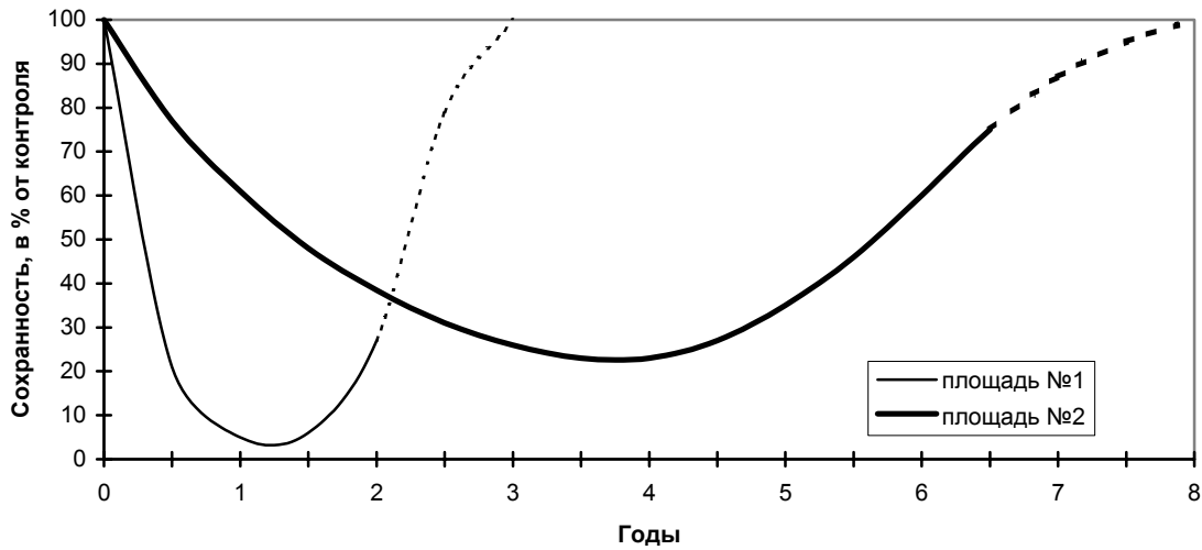
Рис. 8. Дegradационно-восстановительные процессы относительного обилия животных в различных сообществах мелких млекопитающих с нефтезагрязненных территорий средней степени.
